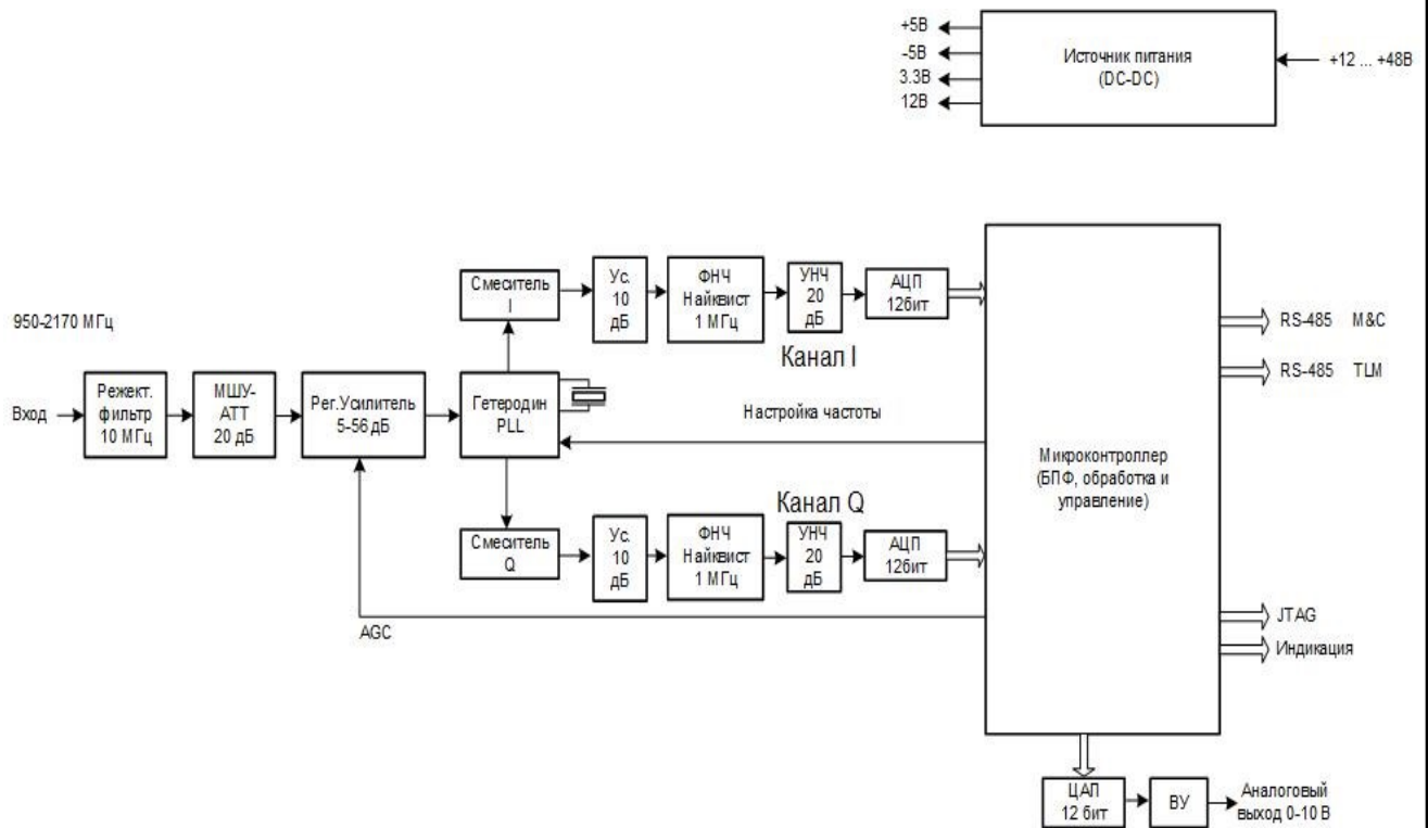
Рисунок 1.4.1 - Функциональная схема приемника сигнала наведения ЦПСН
